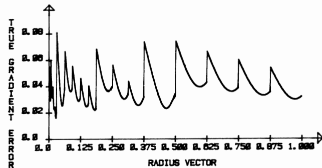
Fig 4.3 Gradient error
